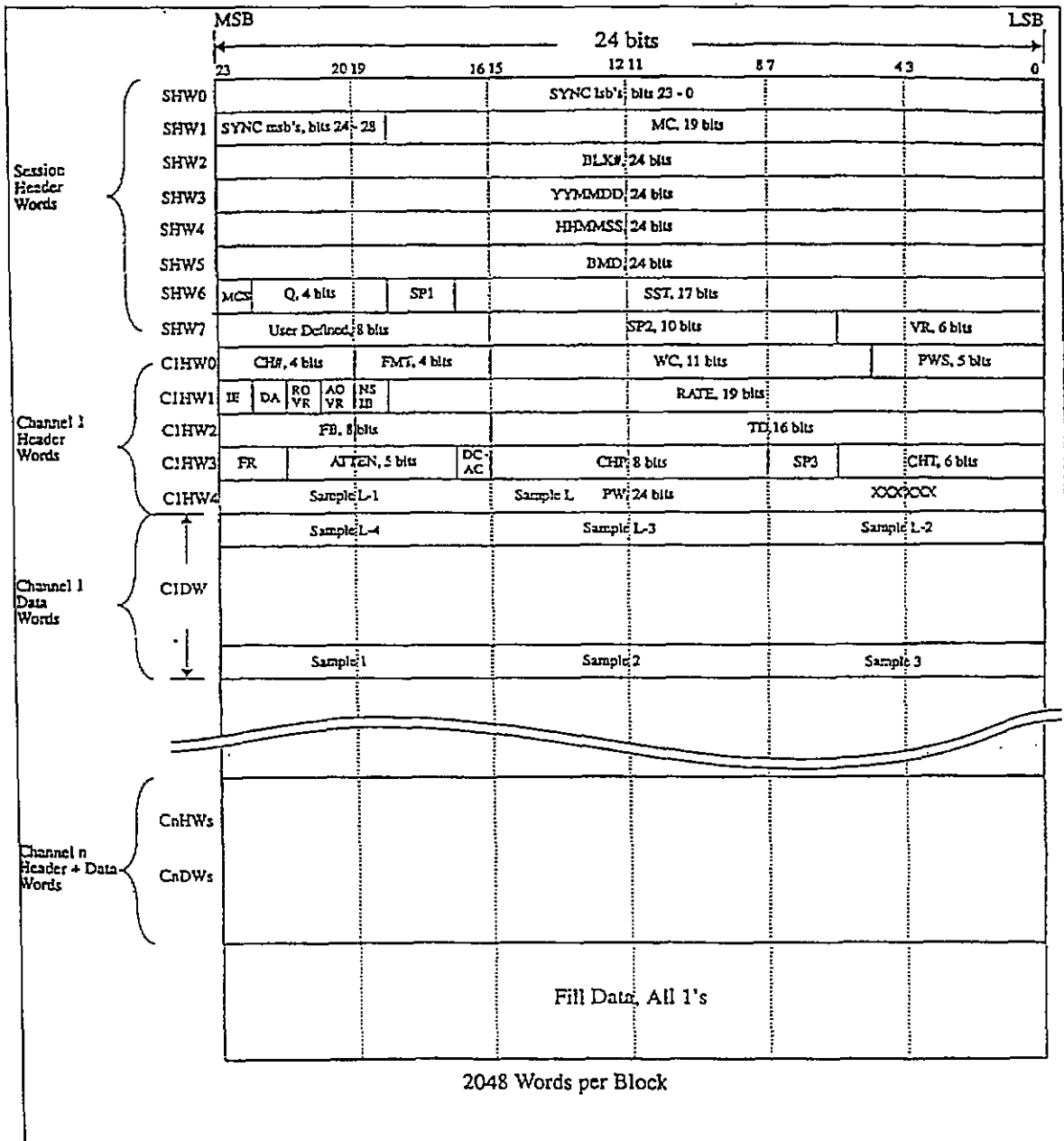
Figure 6-8. ADARIO data format.
